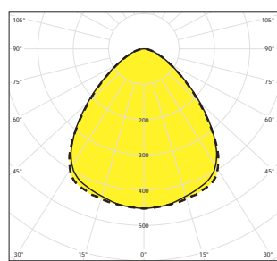
LARO20-S-4K, IP20
