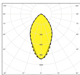
LARO20-H-4K, IP20
