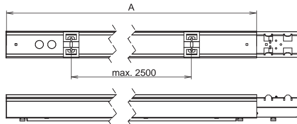
LARO20-LED
